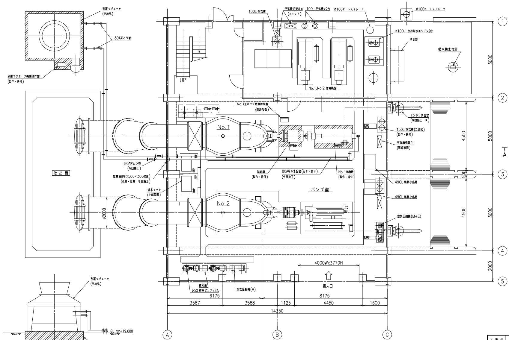
配置断面図 (別置フジエータ部)
