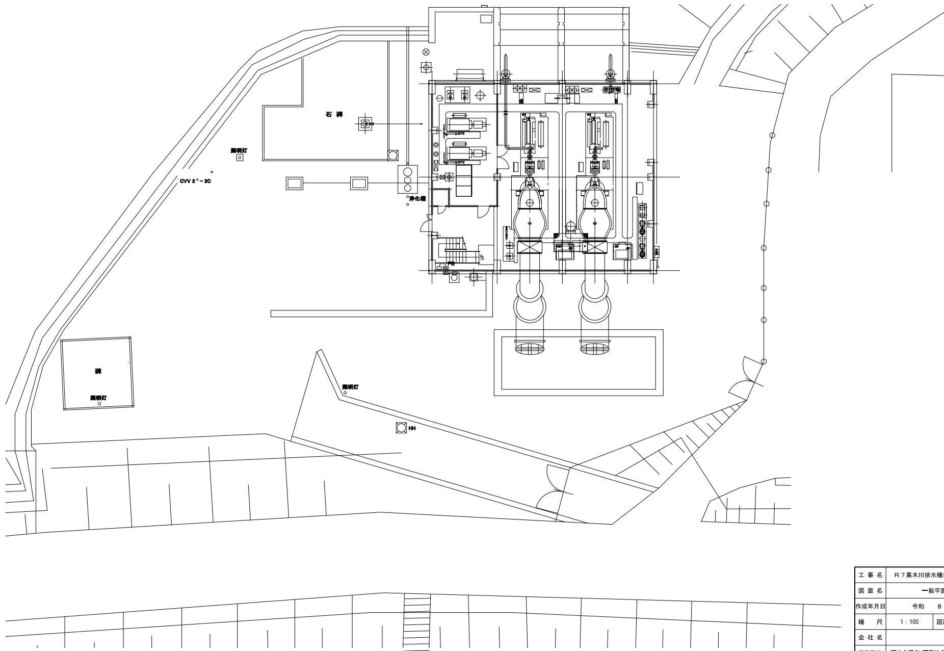
一般平面図 (既設) S = 1 / 100
