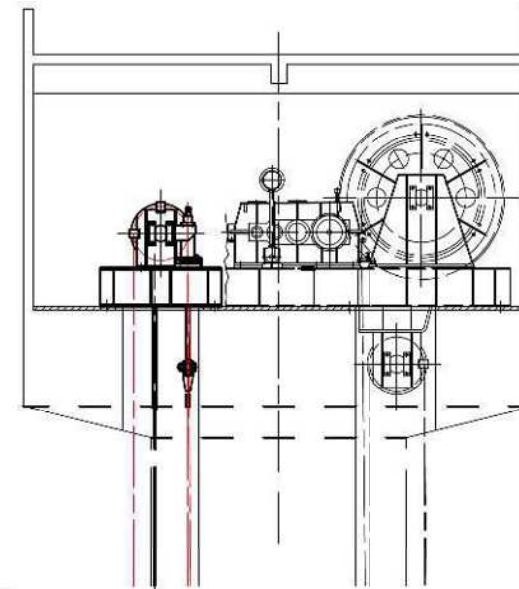
正面図 (S=1:40)
