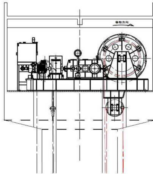
正面図 (S=1:40)
