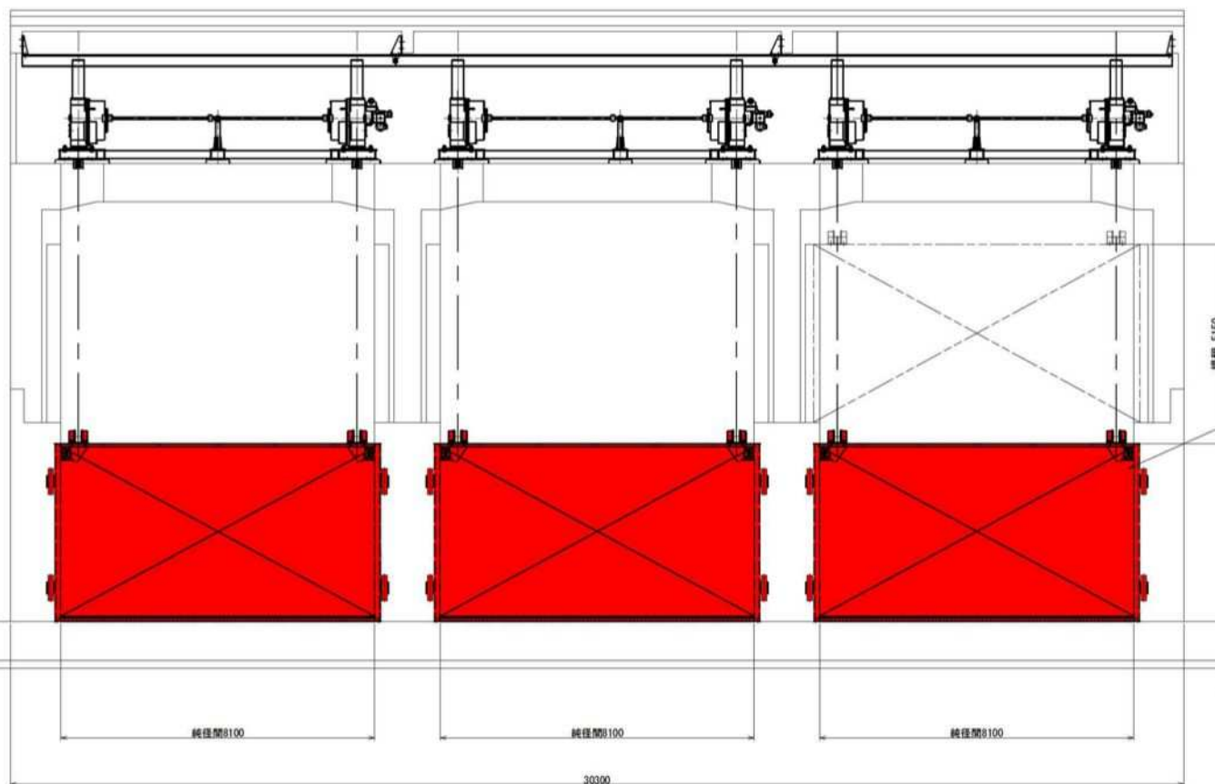
正面図
