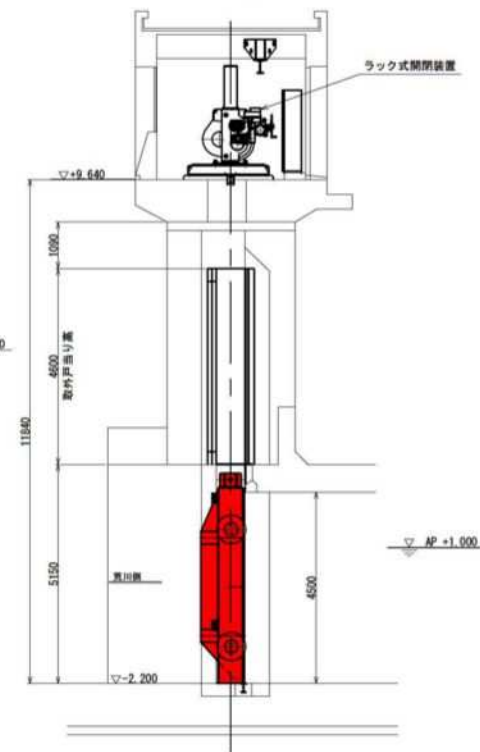
縦断面図
