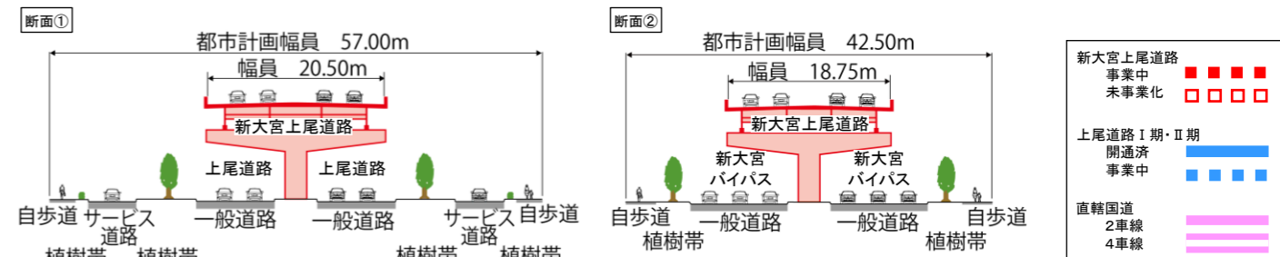
標準断面図 (計画)
