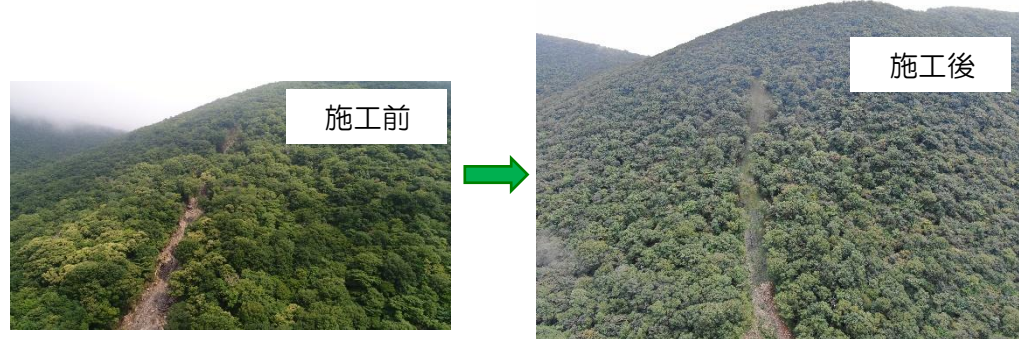
渓間工（荒廃渓流の復旧工事：コンクリート谷止工） 施工地：渋川市
