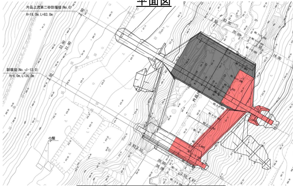
平面図
