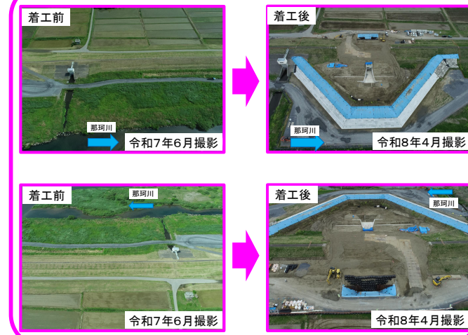
① 常陸大宮市大場地区（那珂川左岸33.5k付近）
