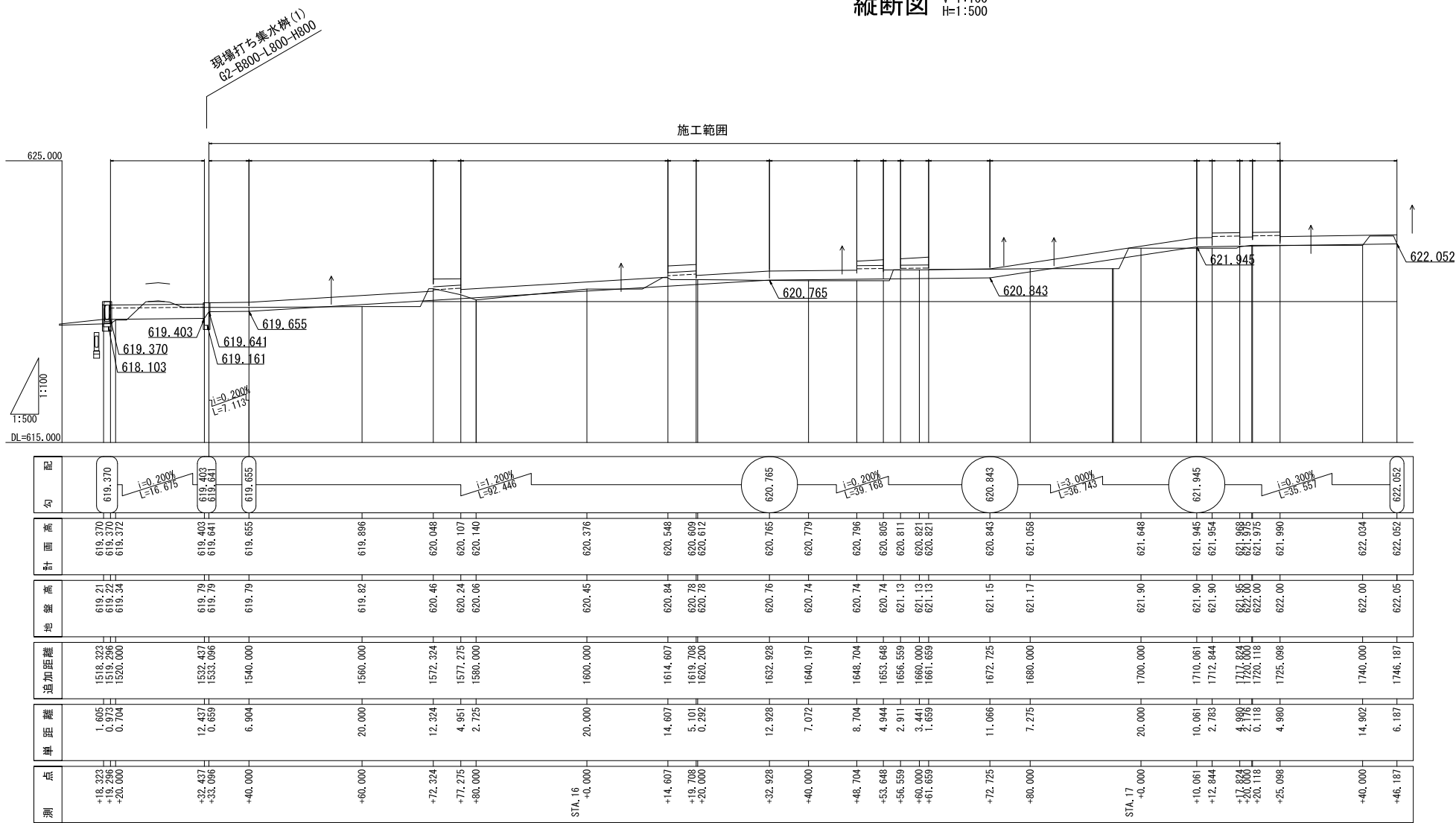
縦断面図 V=1:100 H=1:500
