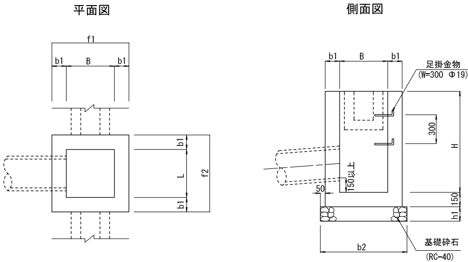
現場打ち集水枡 (1) ~ (3) G2型集水ます
