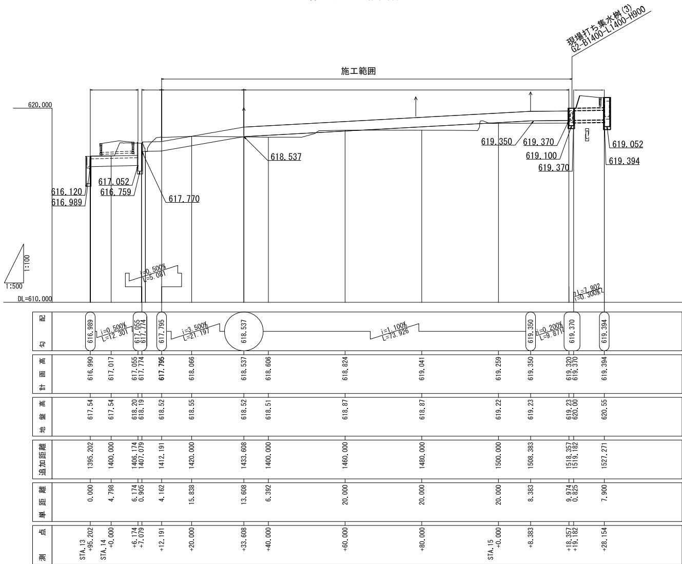
縦断面図 V=1:100 H=1:500
