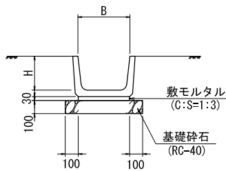
プレキャストU型側溝 (1) (2) (BF1)
