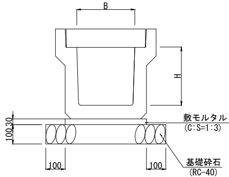
プレキャストU型側溝(2)(3) S=1:10
