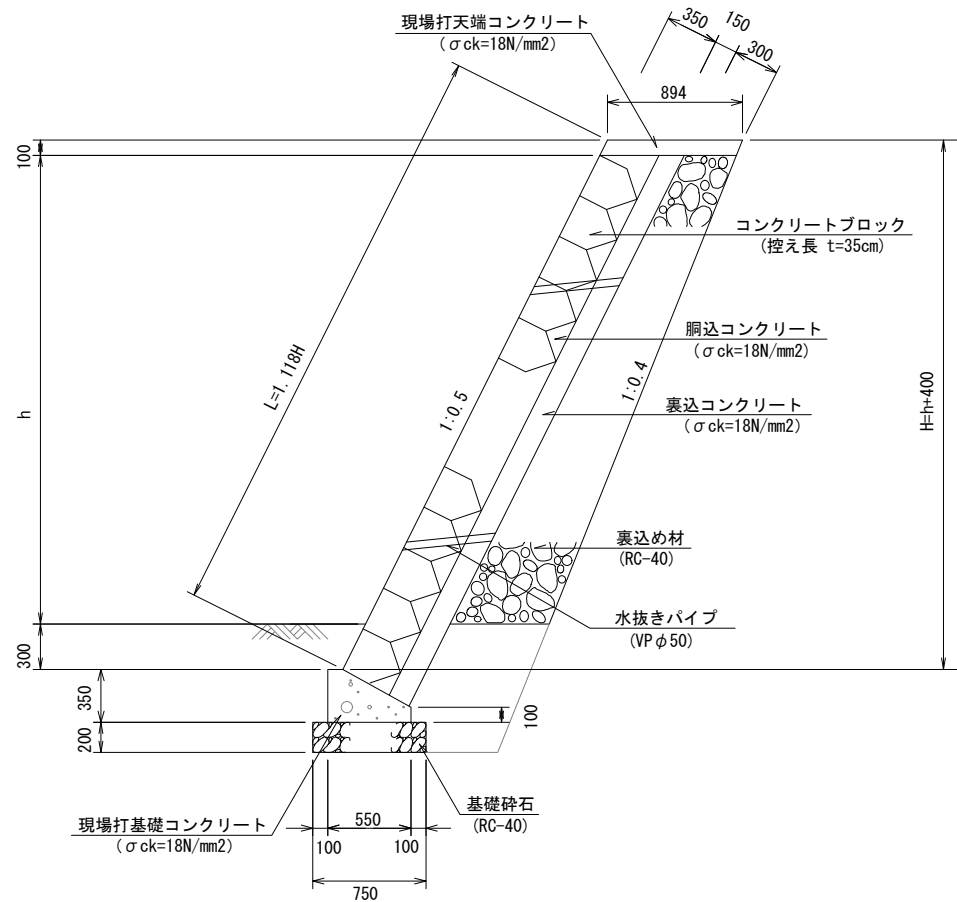
コンクリート(間知)ブロック積 S=1:25
