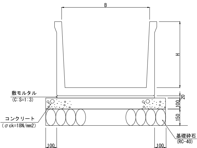
プレキャストU型側溝(4)(5) S=1:10
