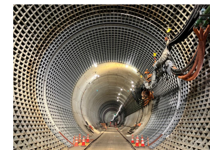
写真⑨：機内覆工完了
