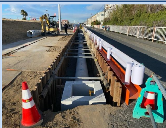
側溝を施工しています。 (令和8年1月)
