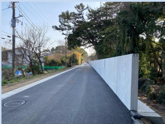
舗装を施工しています。 (令和8年2月)
