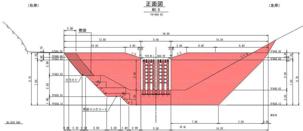
砂防堰堤構造一般図 S=1:100
