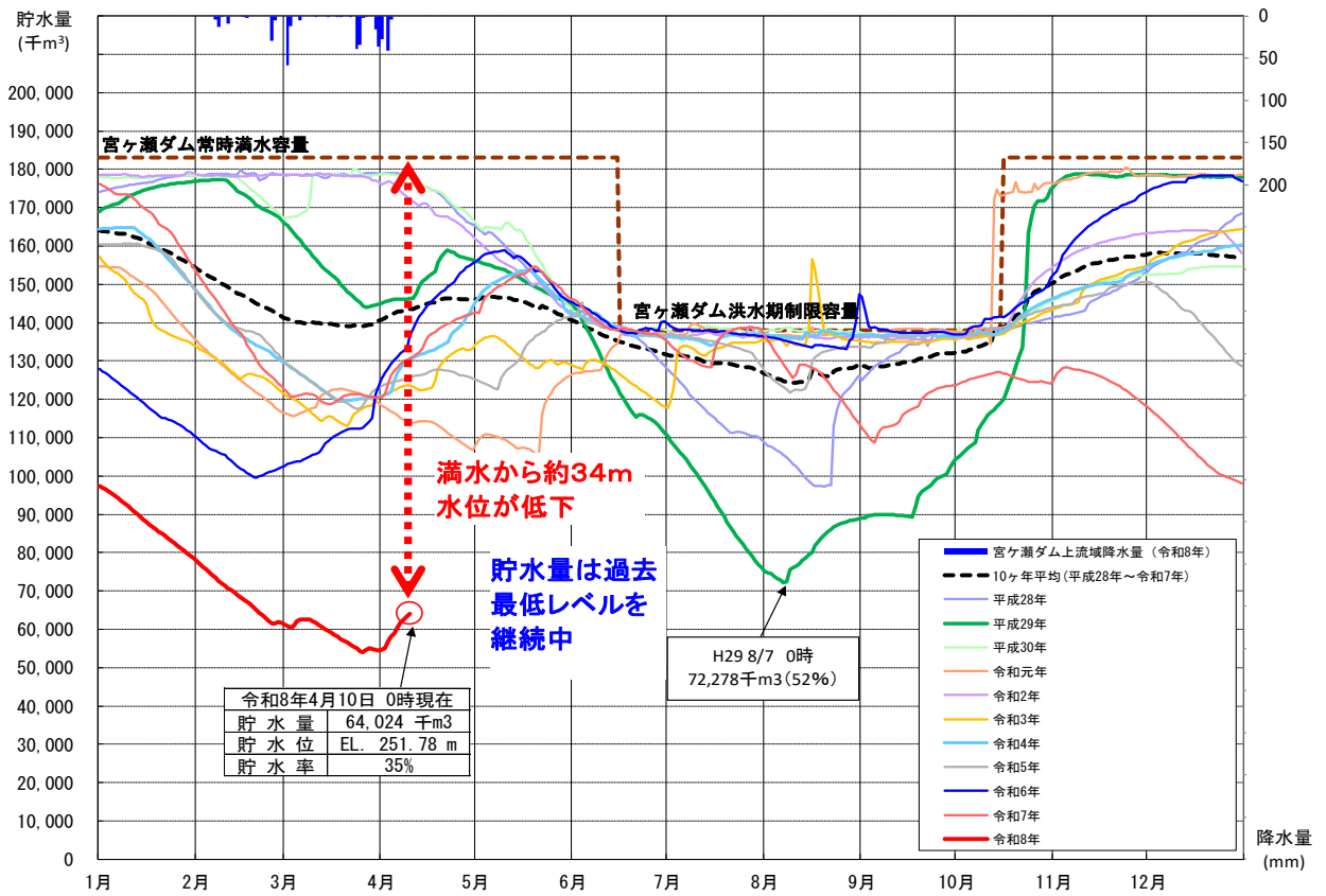
図－2 宮ヶ瀬ダム貯水量図
