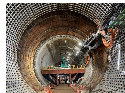
写真⑦：2次解体完了
