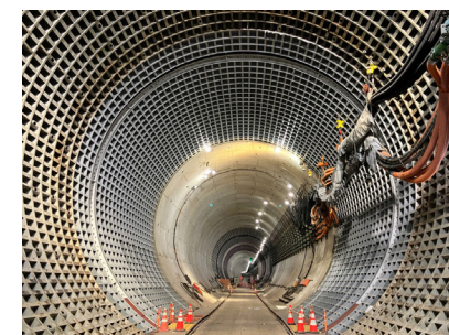
写真⑨：機内覆工完了
