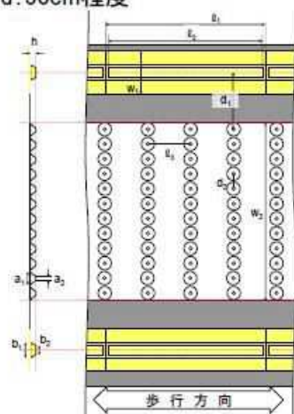
踏切内誘導表示の構造
