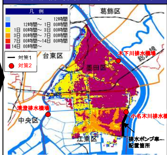
浸水継続時間図[対策1+対策2]
