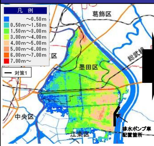
最大浸水深図[対策1]
