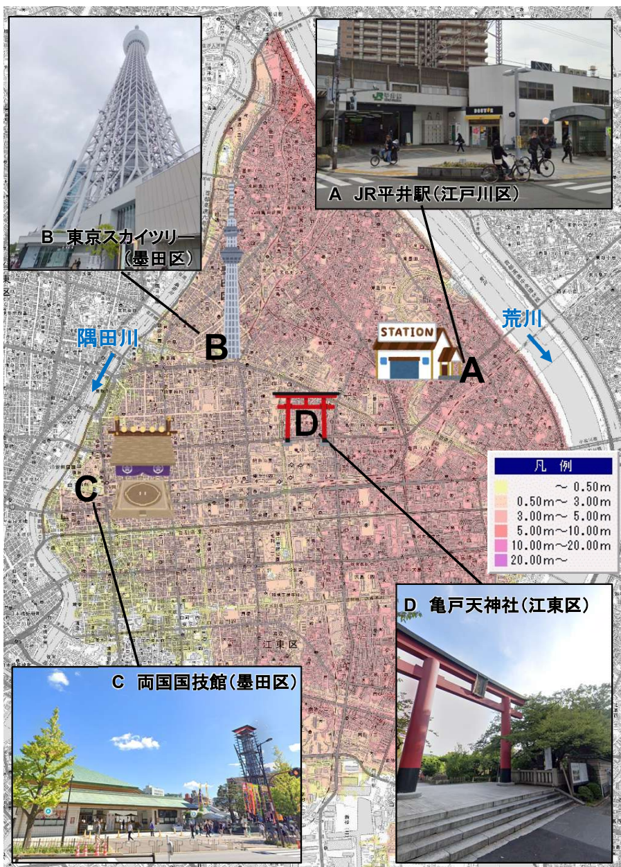
荒川3D洪水浸水想定区域図(下流域) ※(A)JR平井駅
