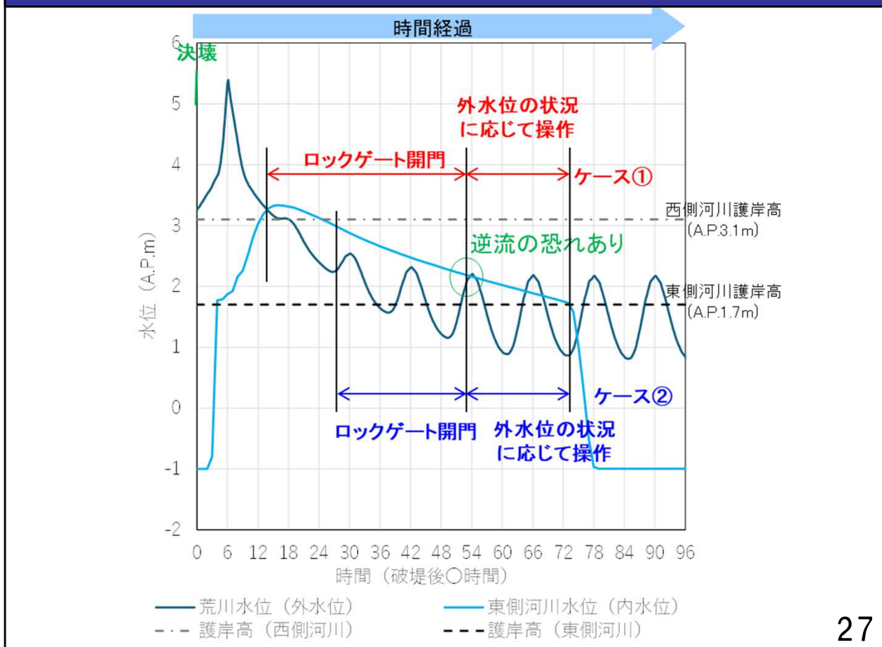
検討における荒川ロックゲートの操作状況
