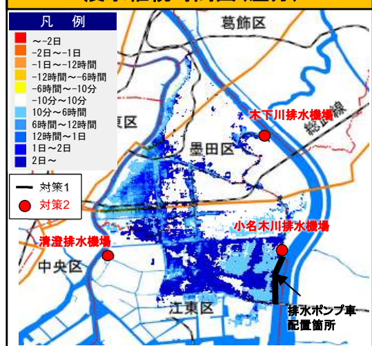
浸水継続時間図(差分)
