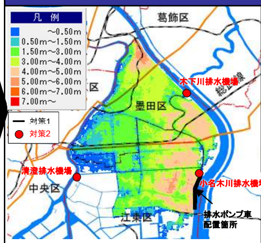
最大浸水深図[対策1+対策2]
