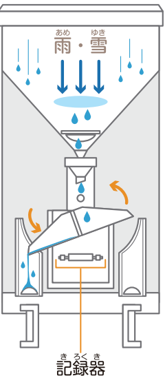
転倒ます型雨量計
