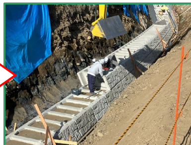
護岸ブロックを設置しています
