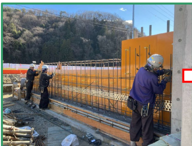
用水樋管(中流部)の型枠を組み立てています
