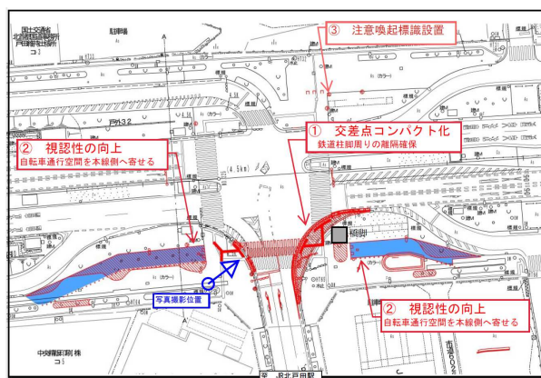
【工事概要図】
