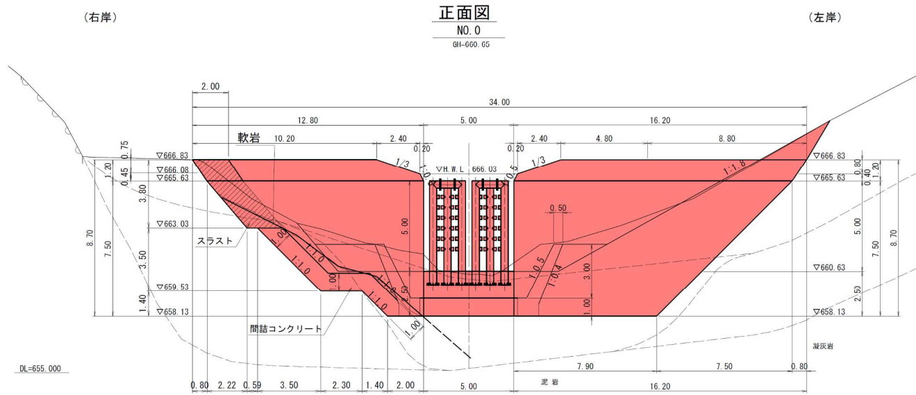
砂防堰堤構造一般図 S=1:100
