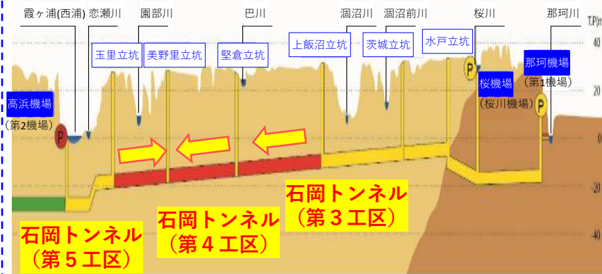
シールドマシンの掘進方向
