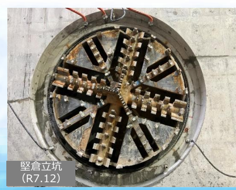
3工区シールドマシン到達
