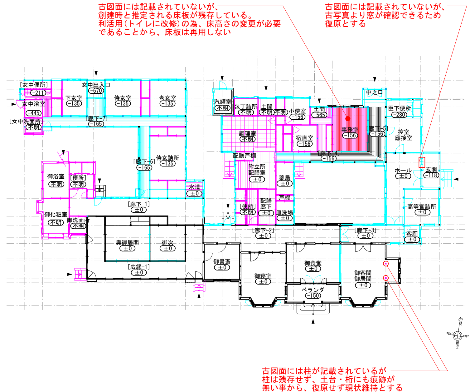
創建時平面図
