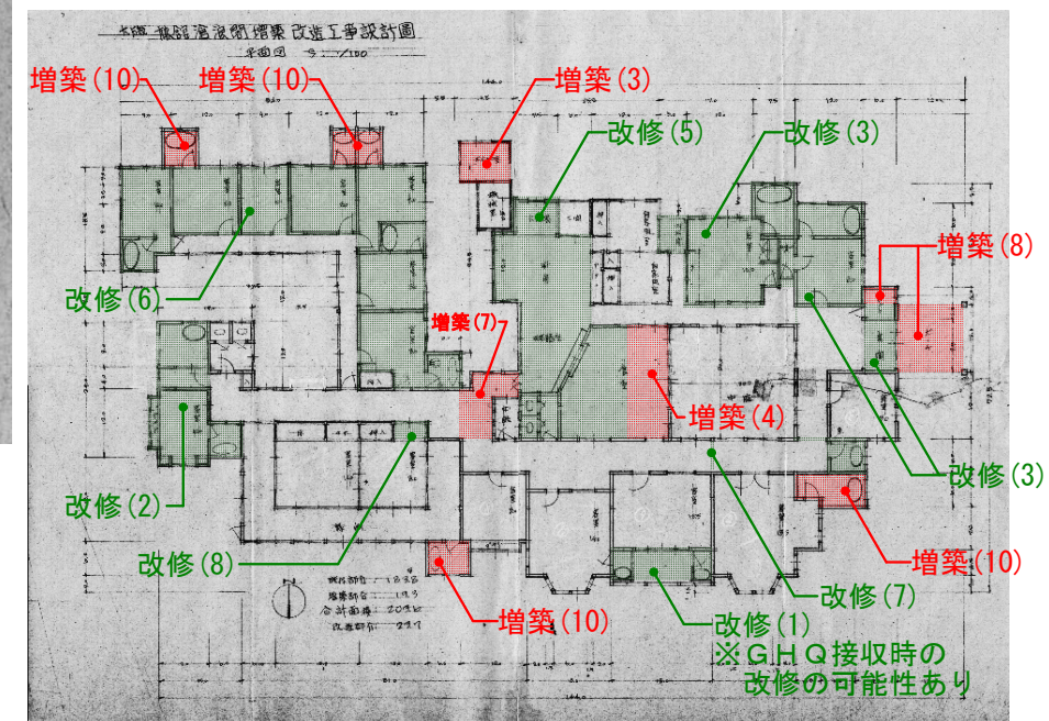
D 大磯旅館滄浪閣平面図(変遷表では「図2」と記載) 作図年：昭和26(1951)年から同30(1955)年(推定) [大磯町立図書館所蔵]
