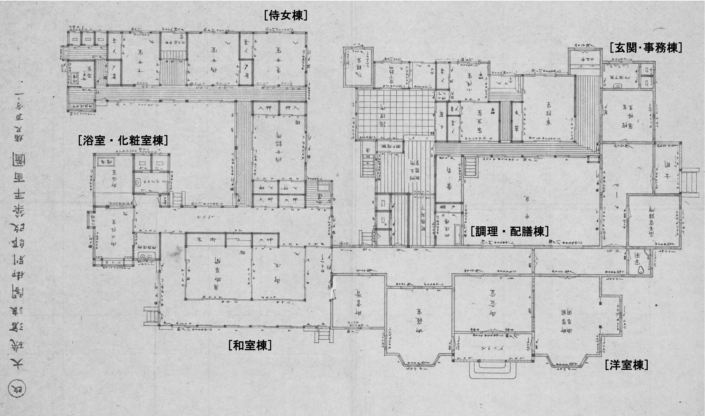
A 改 大磯滄浪閣御別邸改築平面図（変遷表では「図1」と記載）
