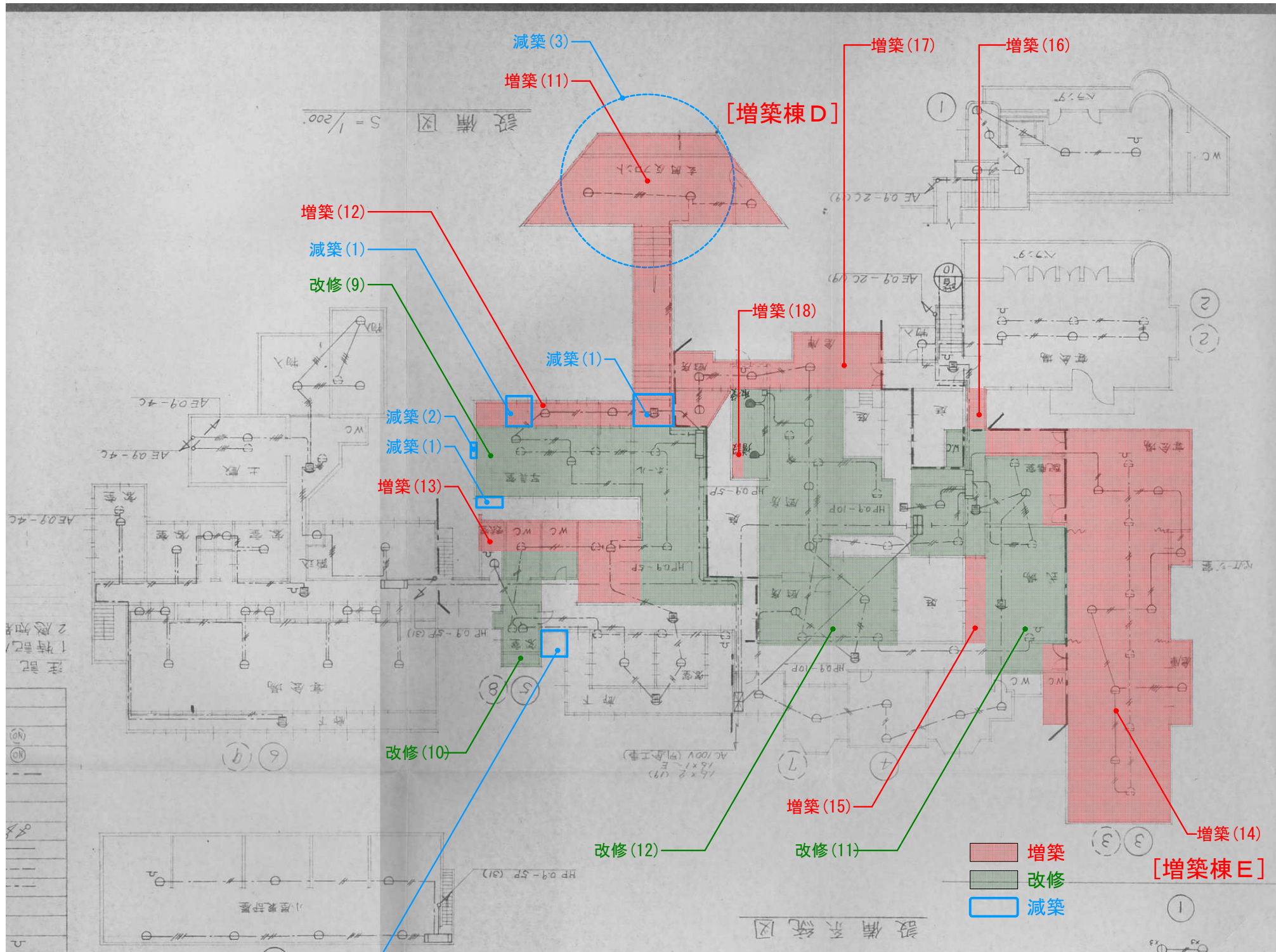
J 西武鉄道株式会社「消防要設備着工届出書 設備図」(変遷図では「図4」と記載) 作図年：昭和59(1984)年(推定) [国土交通省所蔵]
