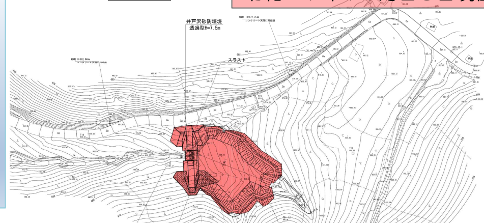
平面図
