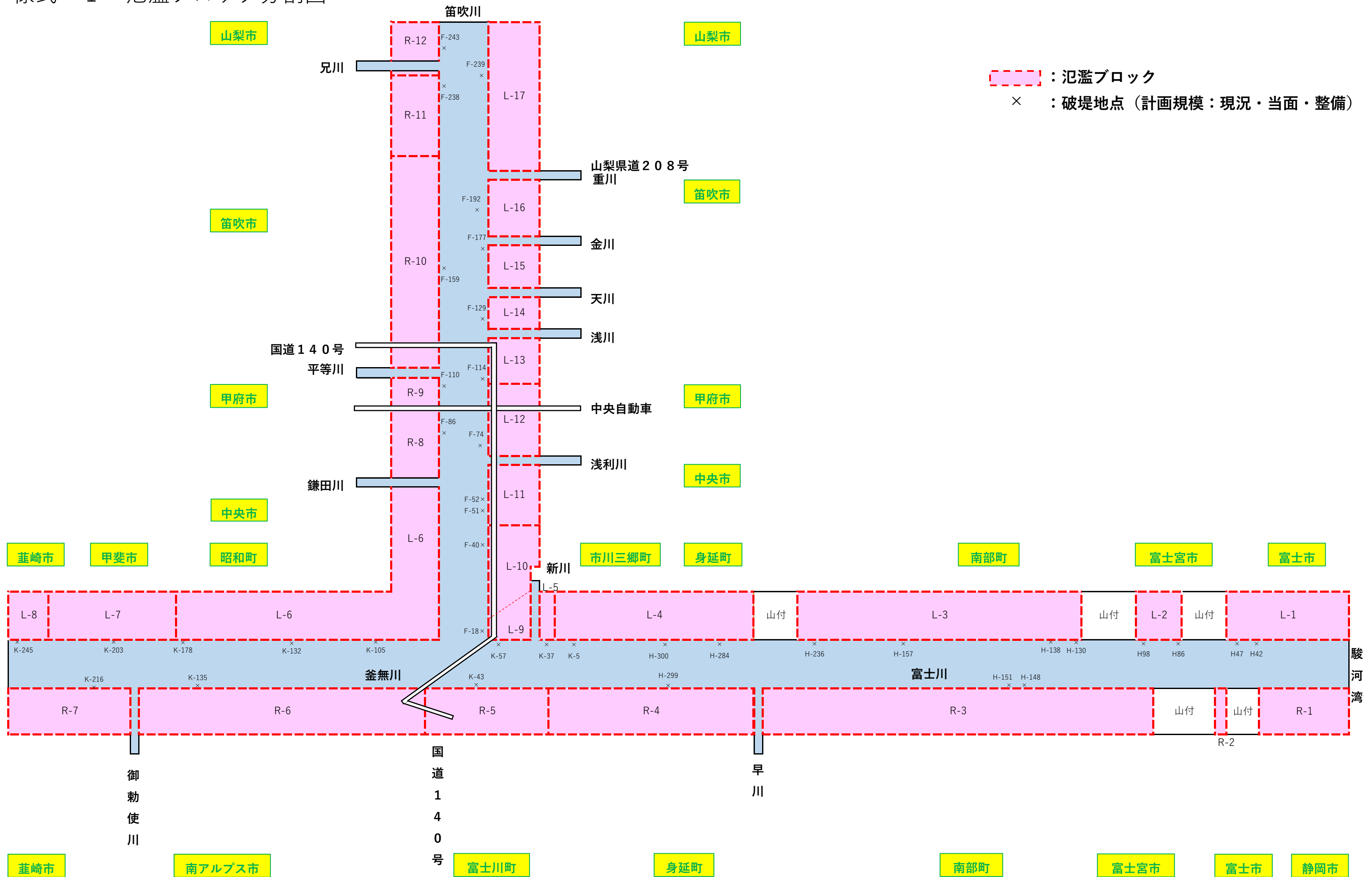
様式－１ 氾濫ブロック分割図
