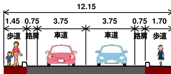
【現況断面図】 (単位: m)
