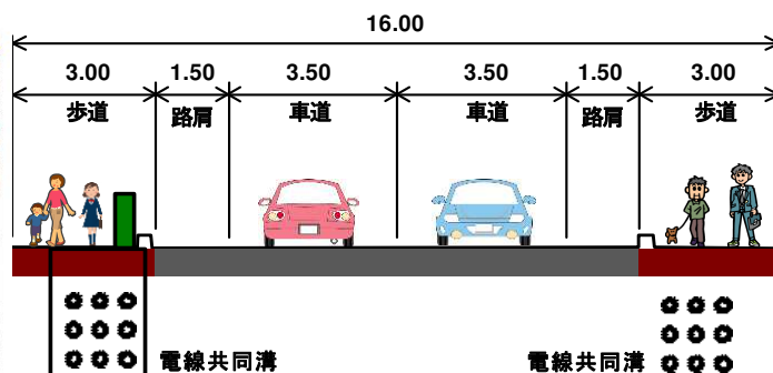
【計画断面図】 (単位: m)
