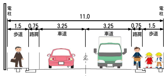
【現況断面図】 (単位：m)
