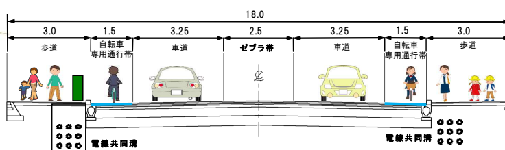
【計画断面図】 (単位：m)
