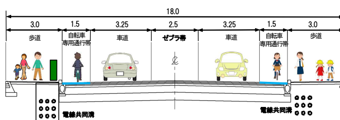
【計画断面図】(単位: m)
