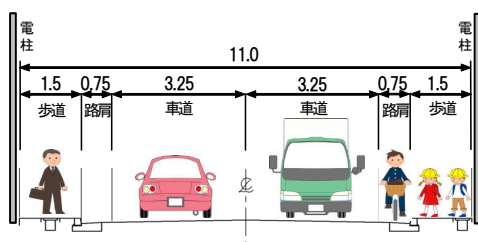
【現況断面図】(単位: m)
