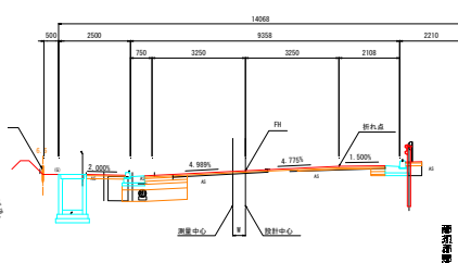
■線形改良箇所 断面図
