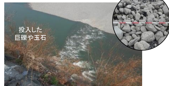
巨礫や玉石配置の実例 施行後には大規模な瀬淵環境が形成されている
