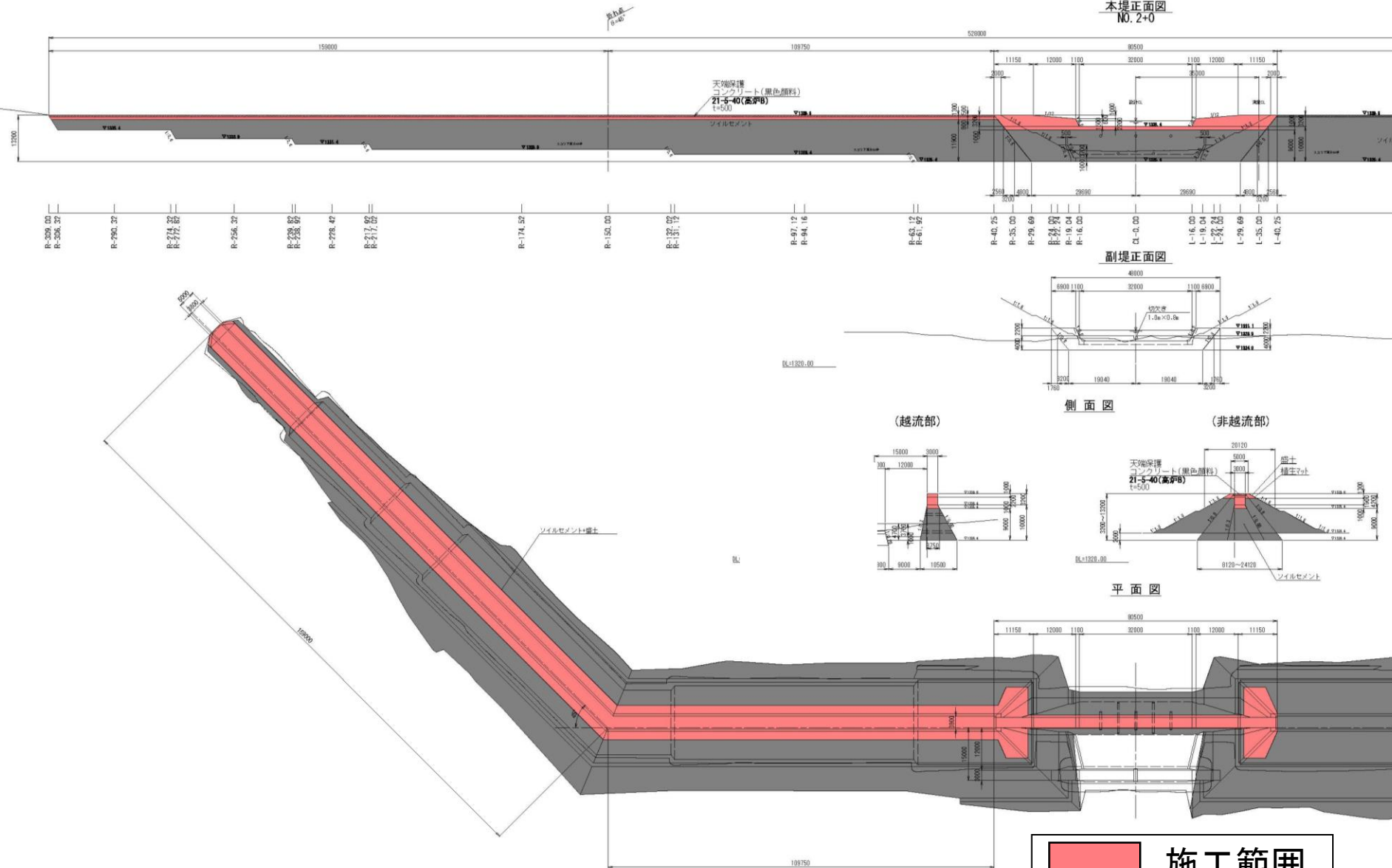
砂防堰堤一般図 S=1:500 (本堰堤右岸側)
