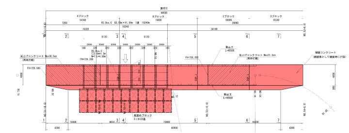
正面図
