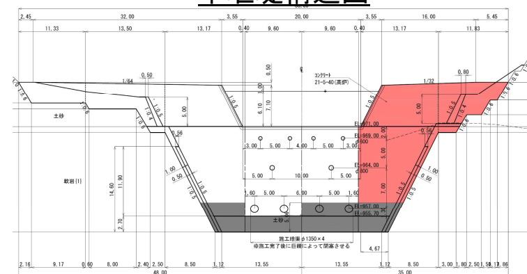
副堰堤構造図
