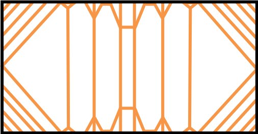
大火打ち式土留め支保工
