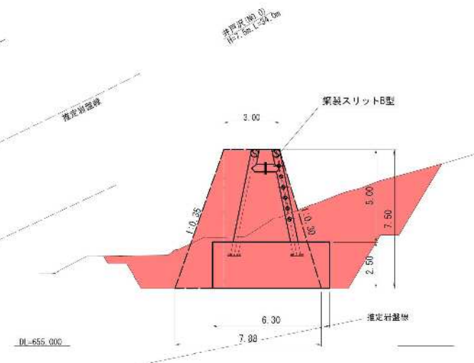
非越流部側面図
