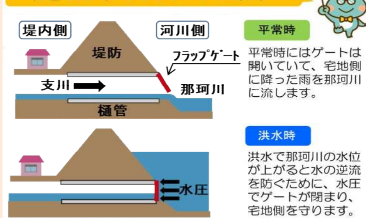
樋管とは（フラップゲートの場合）
