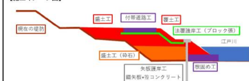
【施工イメージ図】
