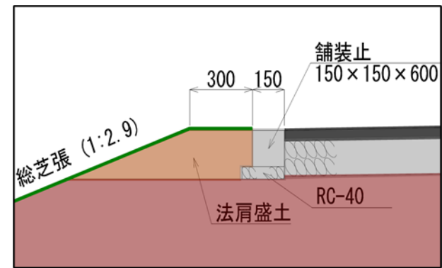
従来の堤防法肩構造
