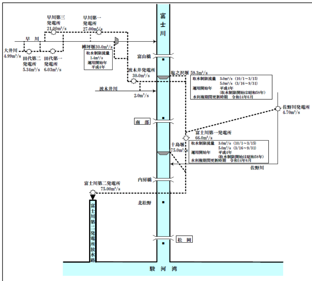
図7 富士川中下流部の発電系統模式図
