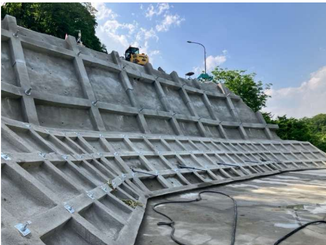
2段目法面:法枠工・鉄筋挿入工完了状況
