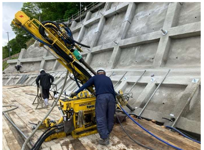
2段目法面:法枠工・鉄筋挿入工施工状況
