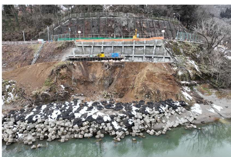
1段目法面:法枠工・アンカー工完了状況
