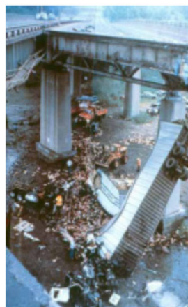
マイアナス橋の崩壊（1983年）
