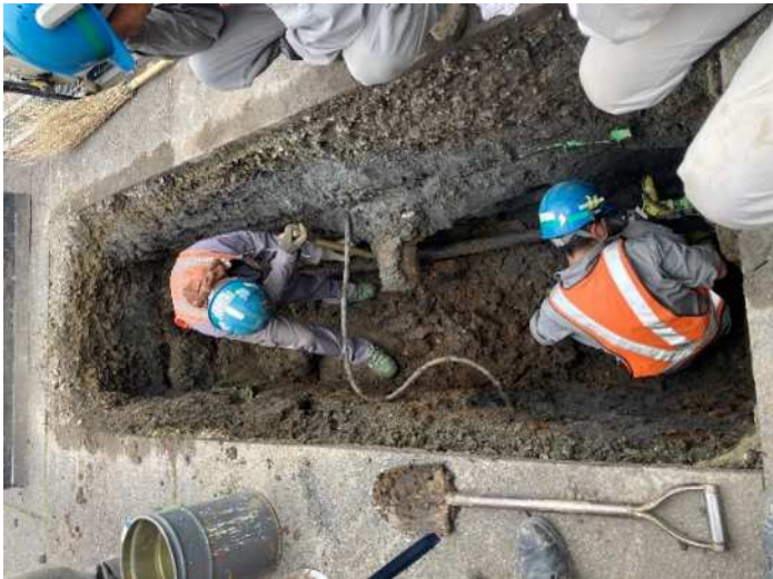
修理状況写真 長野市道（長野県長野市）
