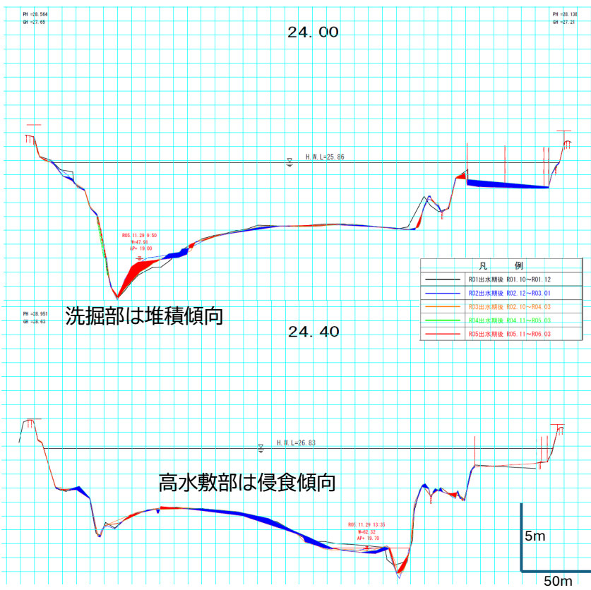
令和元年洪水以降（令和元年～令和5年）の横断面図経年変化
