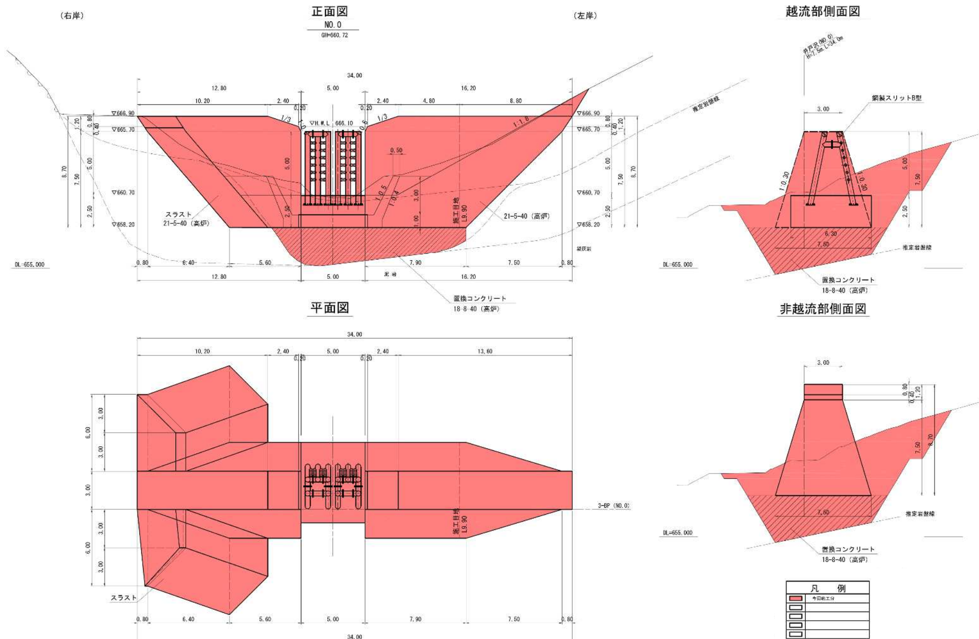
構造一般図 S=1:100
