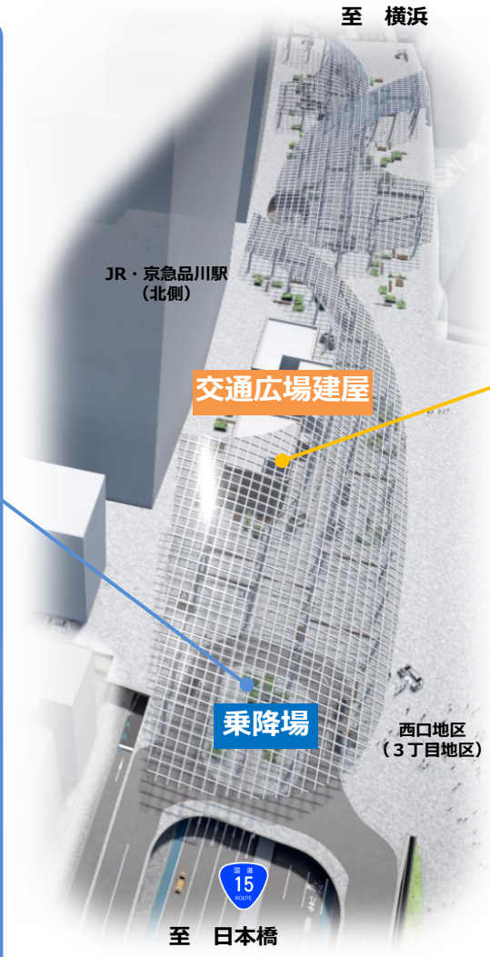
施設配置イメージ (デッキ階)
