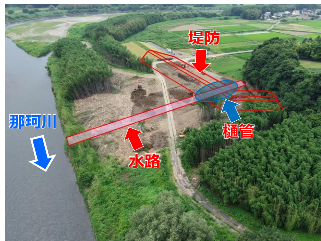
下流側から施工箇所を望む （那須烏山市下境地先）
