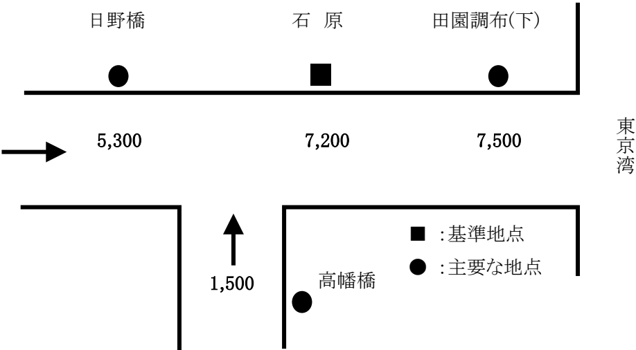
12 図-4-1 主要な地点における整備計画目標流量図(単位:m³/s) 13 14
