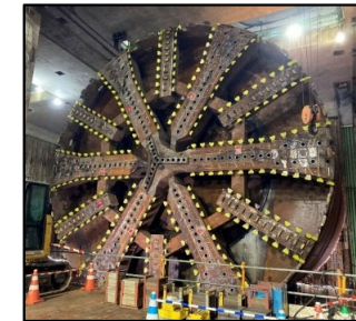
カッタービットの交換（完了）
