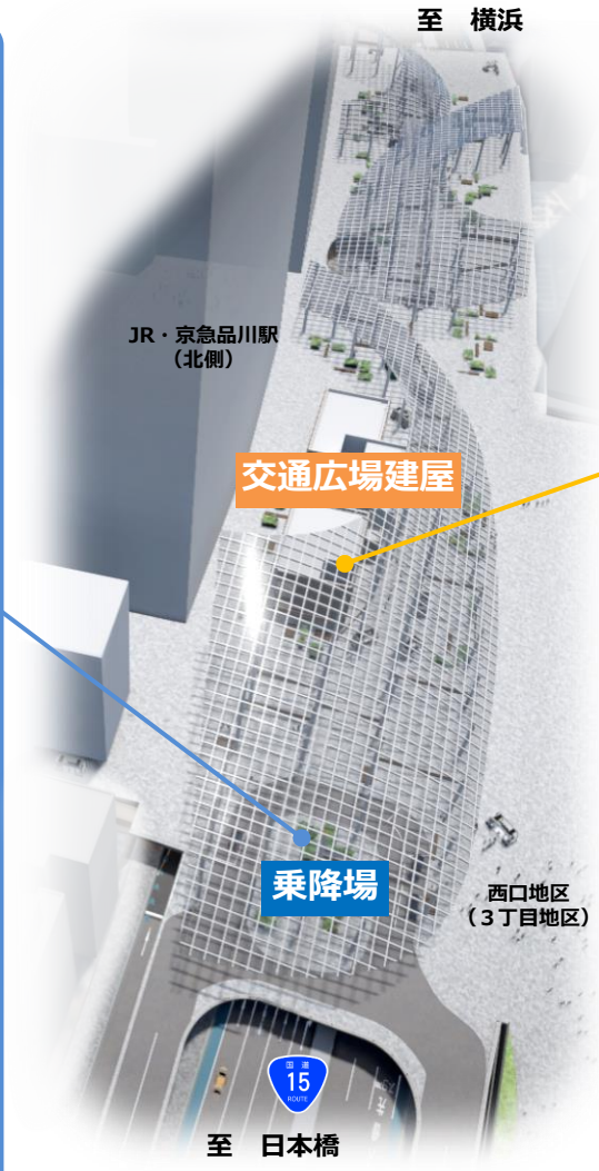
図31 施設配置イメージ（デッキ階）
