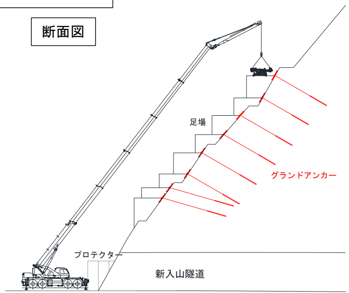
新入山隧道坑口部 法面補強工
